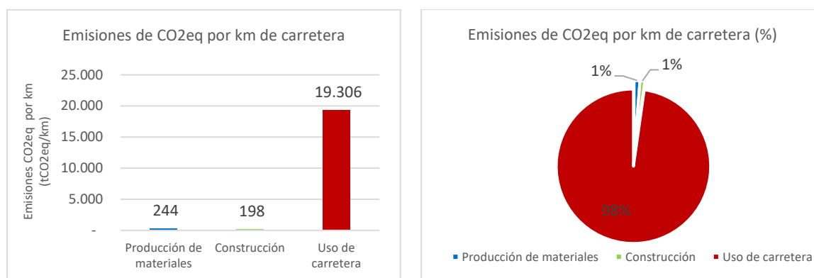
Figura 6: Emisiones de CO 2eq por km para Proyecto Arica- Tambo quemado según fases Fuente: Elaboración propia
