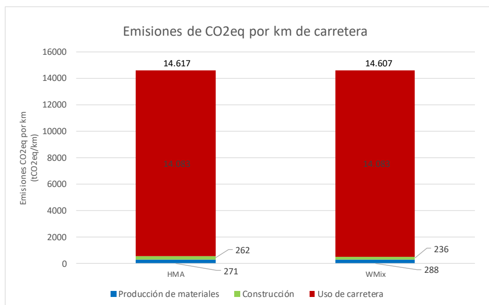
Figura RE 3: Emisiones de CO 2 eq por km para HMA y WMix, según fase Proyecto Lo Orozco-Quilpué Fuente: Elaboración propia
