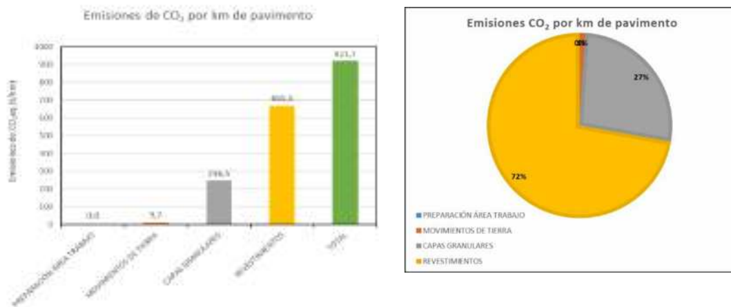
Figura 16: Emisiones de CO 2e según procedimientos de construcción Tramo 3 – Subtramo 1 Proyecto Tegucigalpa- La Venta Fuente: Elaboración propia
