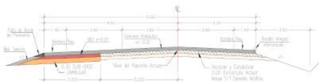
Figura 17: Sección transversal tipo para el tramo Dm 17.500 – Dm 43.900
