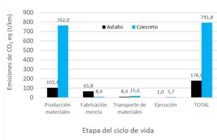
Figura 29: Emisiones de CO 2eq por km según etapa del ciclo de vida para el tramo 2
