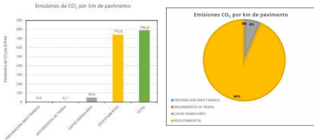
Figura 13: Emisiones de CO 2eq según procedimientos de construcción Tramo 2 Proyecto Tegucigalpa- La Venta (Aldea Santa Rosa – Cerro de Hula) Fuente: Elaboración propia
