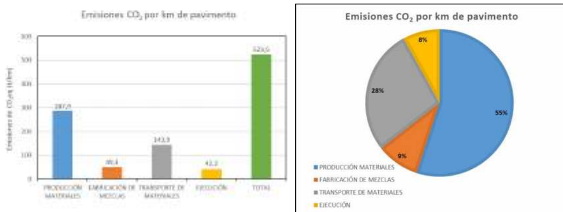
Figura 23: Emisiones totales de CO 2eq según las etapas del ciclo de vida para estructura con mezcla asfáltica tibia (WMix) Fuente: Elaboración propia
